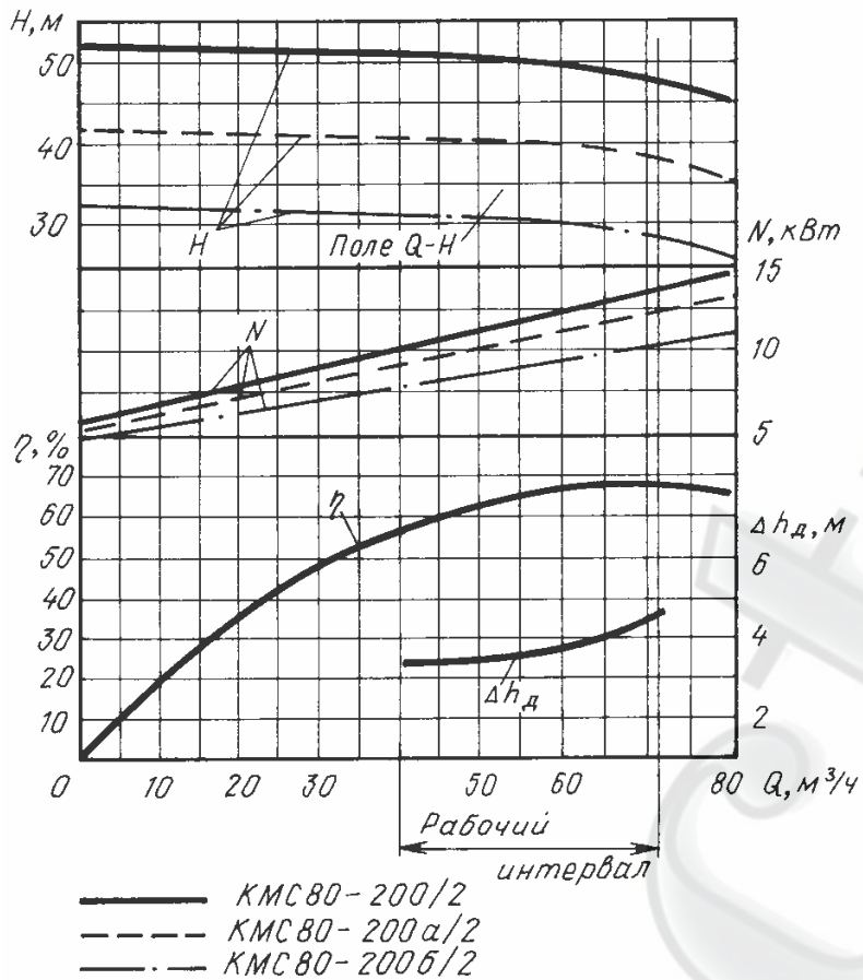
Рис. 2. Характеристики электронасоса КМС80-200/2
